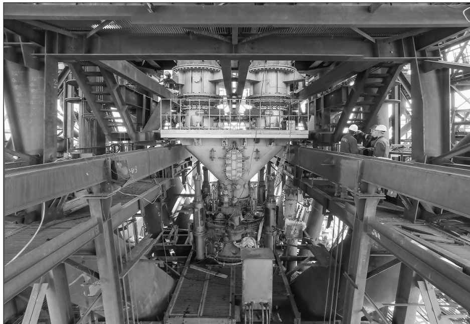
На доменну піч №3 ПАТ "Запоріжсталь" встановили сучасний безконусний завантажувальний пристрій
